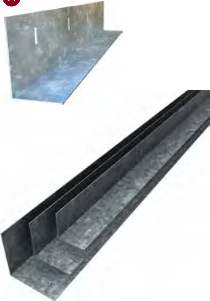
■ RONDO STEEL ANGLES
